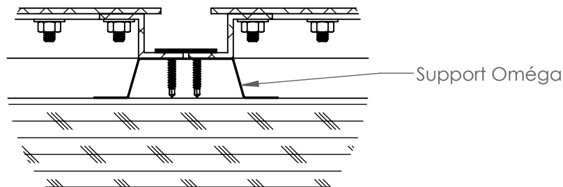
Installation sur Oméga
