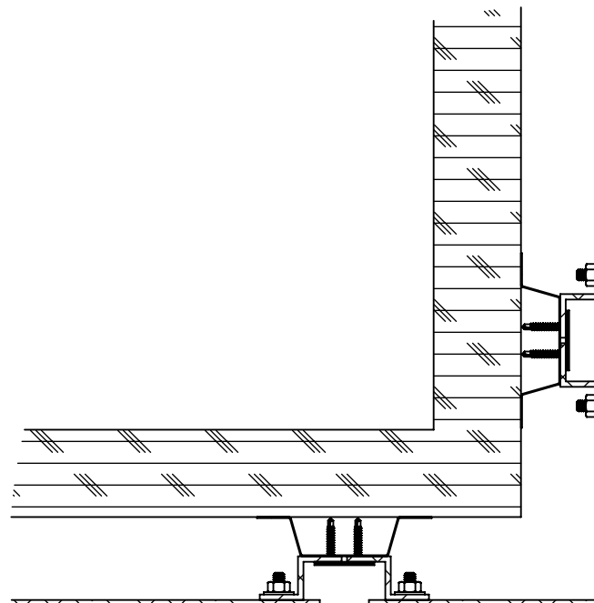
Détails coin extérieur
