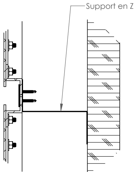
Installation sur Z
