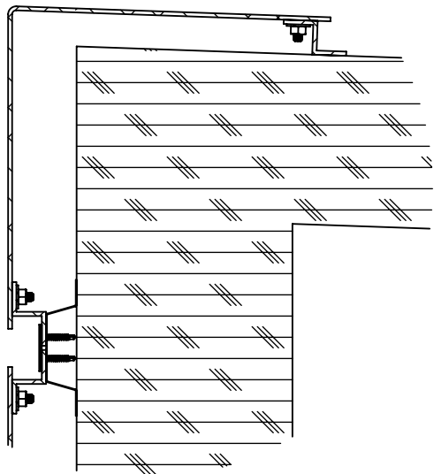
Détails parapet en L
