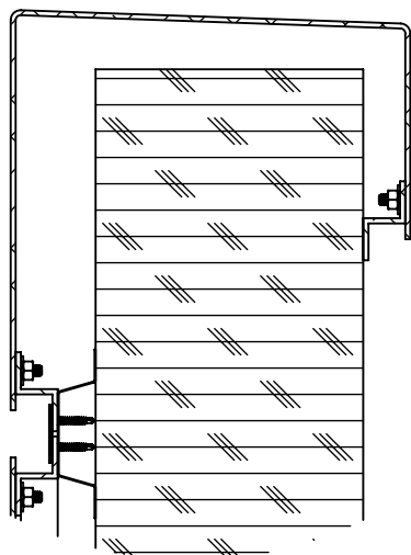
Détails parapet en U
