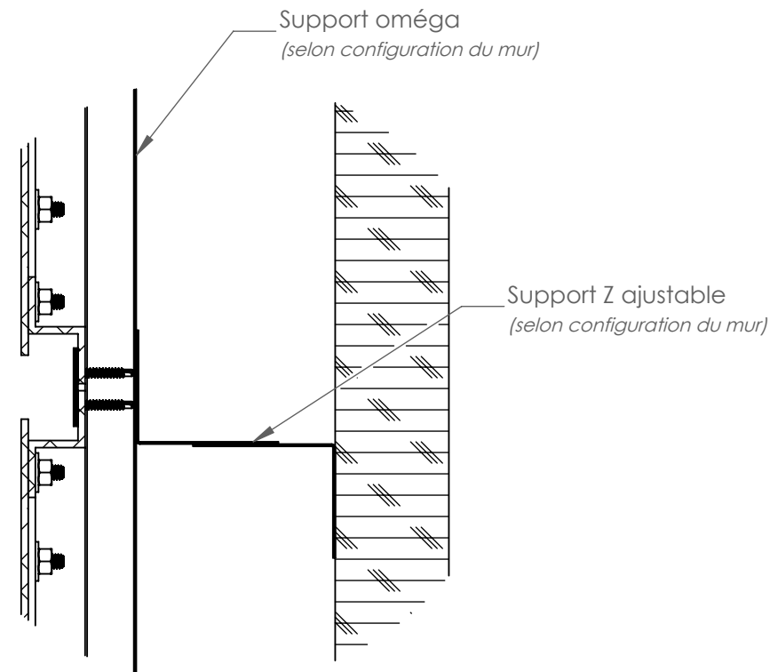
Installation sur Z ajustable (selon configuration du mur)
