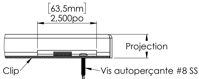
Jonction vue de dessous
