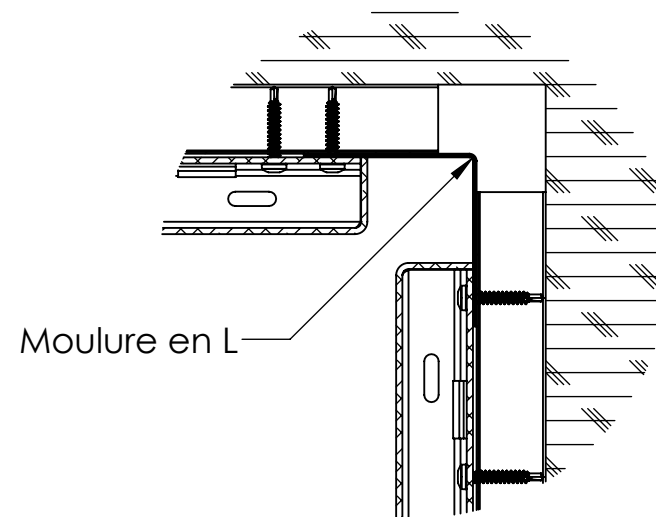
Détail Coin intérieur avec moulure en L
