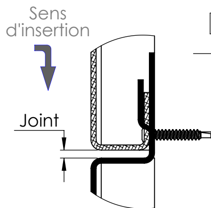
Jonction vue de profil
