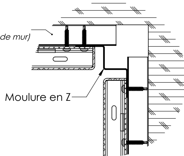
Détail Coin intérieur avec moulure en Z
