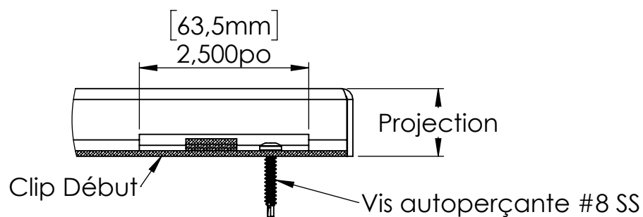
Début vue de dessous
