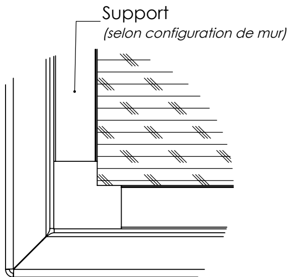
Détail Coin extérieur
