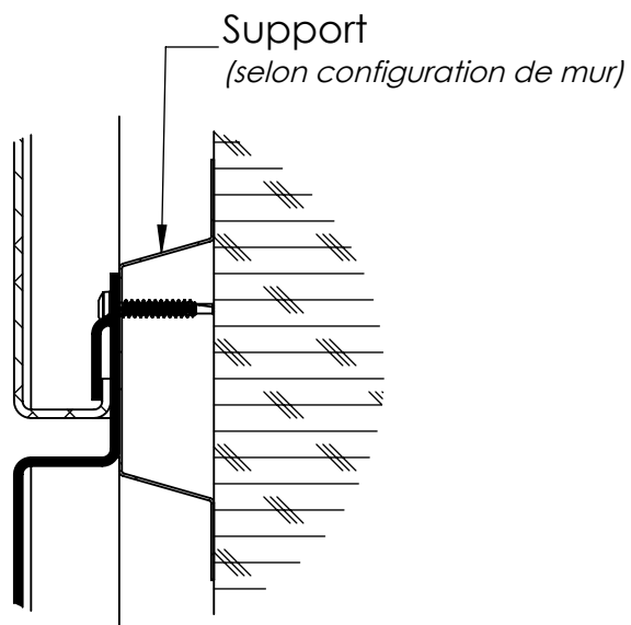
Installation sur Oméga
