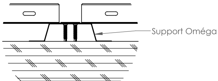
Installation sur Oméga
