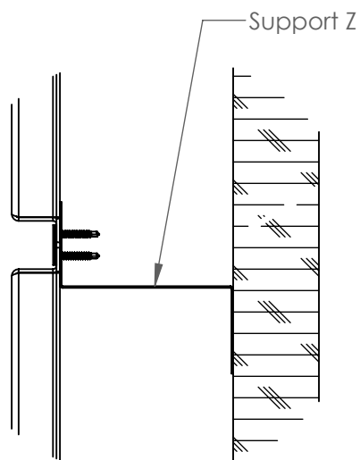
Installation sur Z
