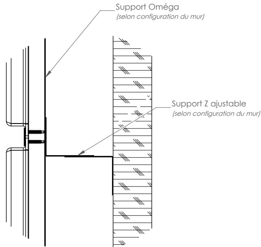
Installation sur Z ajustable
