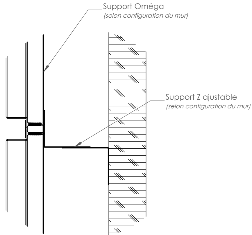
Installation sur Z ajustable
