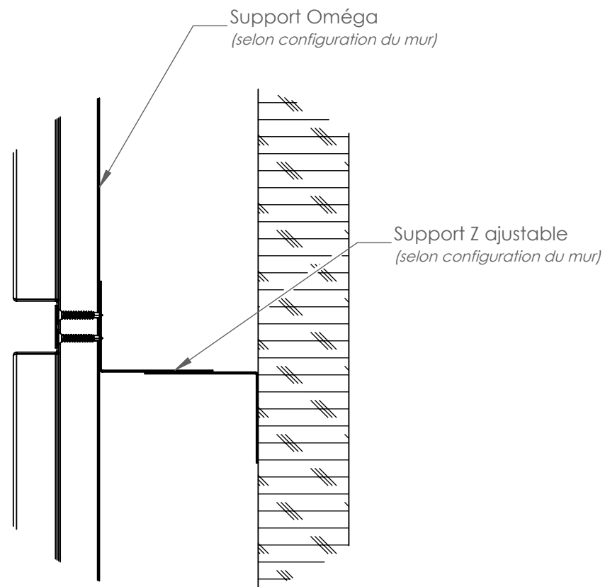
Installation sur Z ajustable
