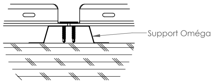
Installation sur Oméga
