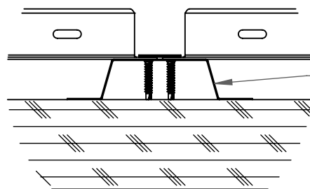
Installation sur Oméga
