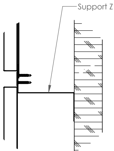
Installation sur Z
