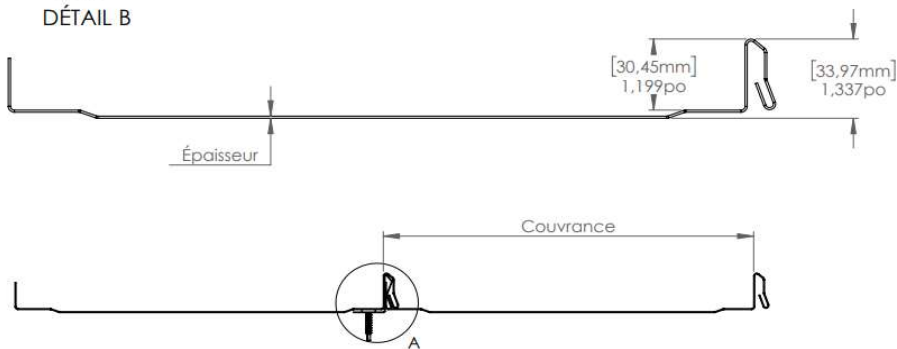
DÉTAIL B
