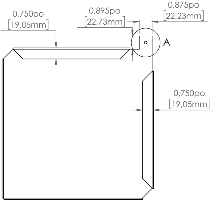
VUE AVANT
