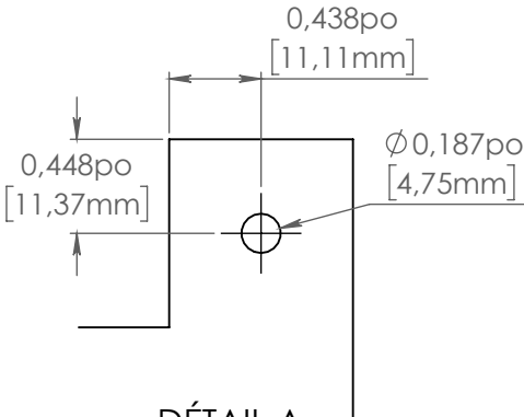
DÉTAIL A ECHELLE 1 : 1
