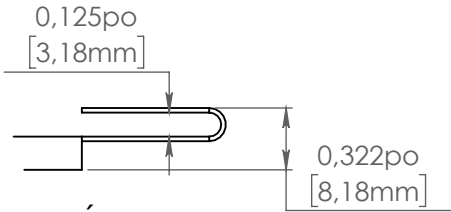
DÉTAIL B ECHELLE 1 : 1
