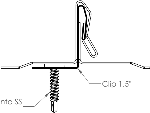
DÉTAIL A ECHELLE 1 : 1
