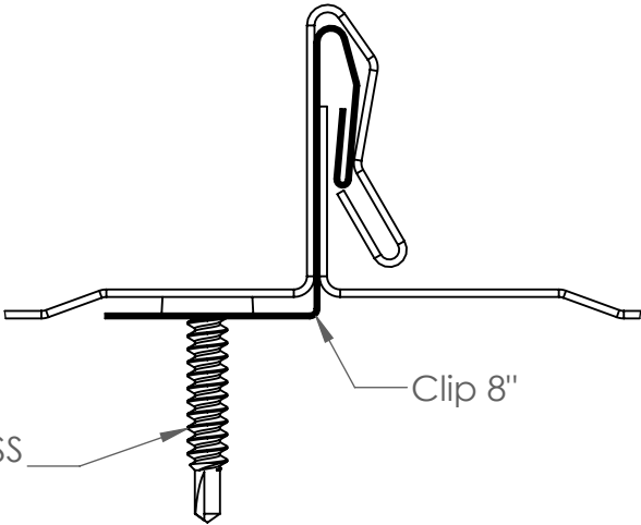
DÉTAIL C ECHELLE 1 : 1
